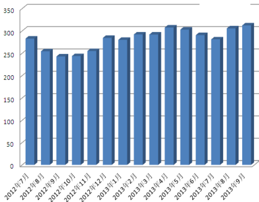
34家优特钢钢厂月产量
