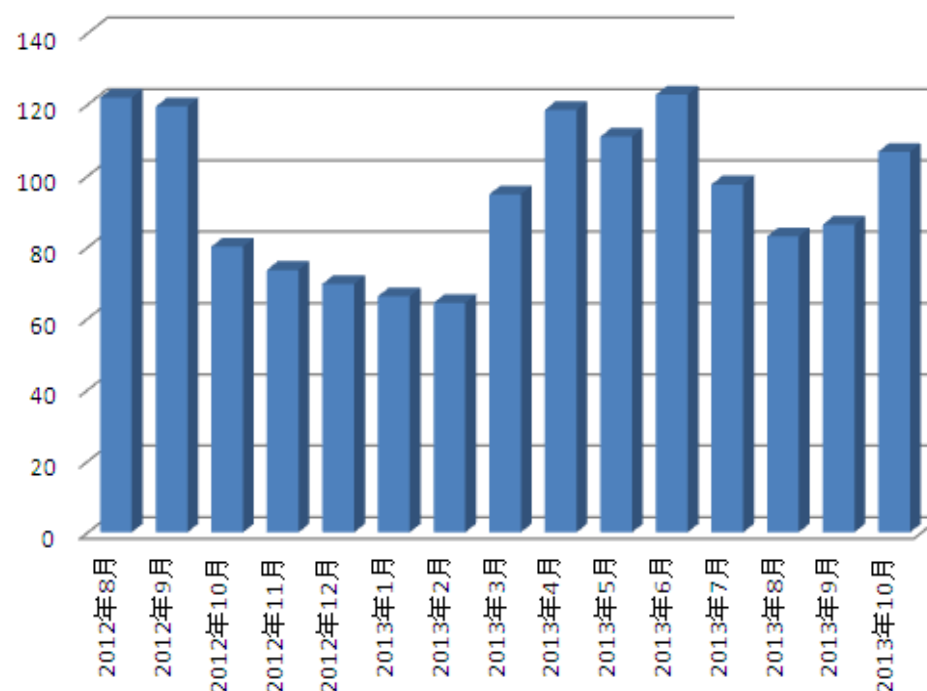
34家优特钢钢厂棒材库存
